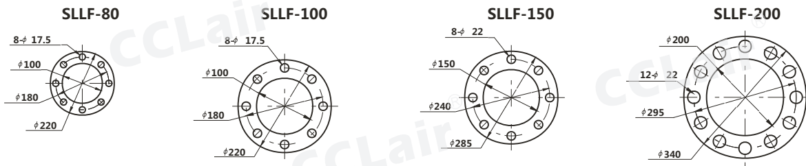
外接法兰连接尺寸
